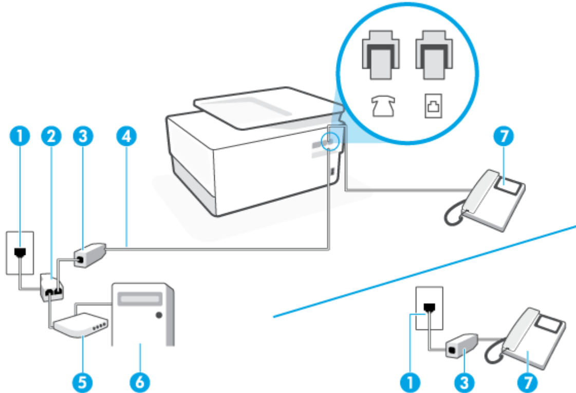
Figura 8-10 Vista posterior de la impresora
