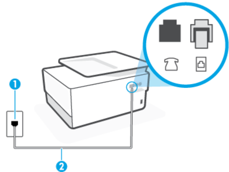
Figura 8-1 Vista posterior de la impresora
