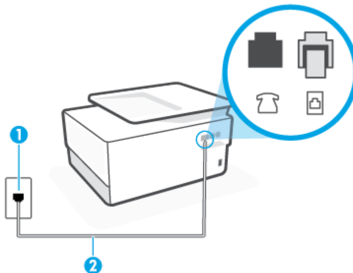
Figura 11-1 Vista posterior de la impresora
