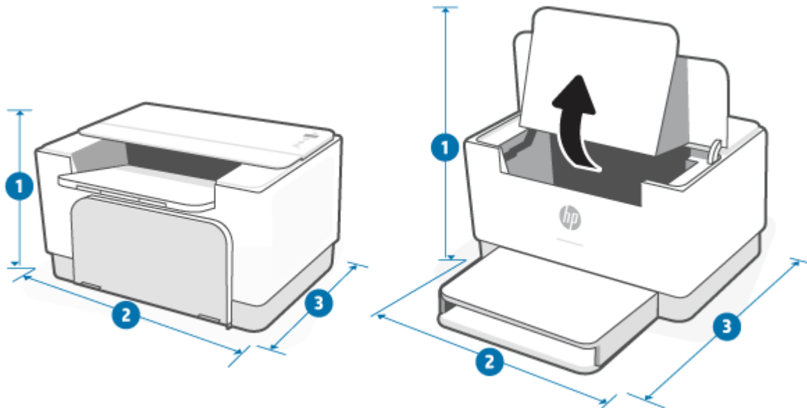
Joonis A-1 Printeri mõõtmed
