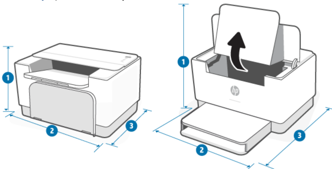
A-1 iliustracija Spausdintuvo matmenys
