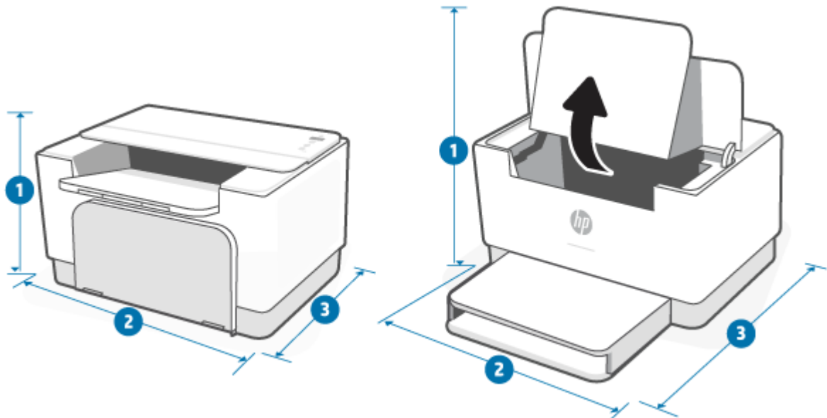
Slika A-1 Dimenzije tiskalnika
