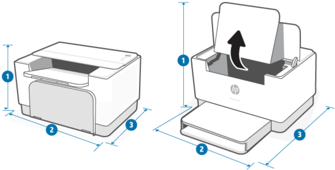
Hình A-1 Kích thước của máy in
