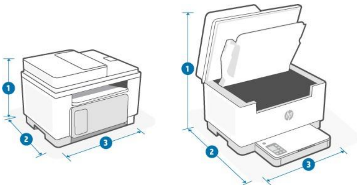
Figura A-2 Dimensioni della stampante (modello sdn/sdw)
