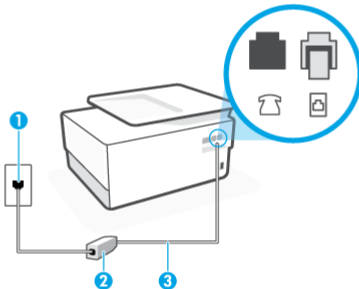
Kuva 8-2 Tulostin takaa
