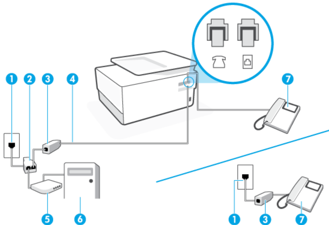
Kuva 8-10 Tulostin takaa
