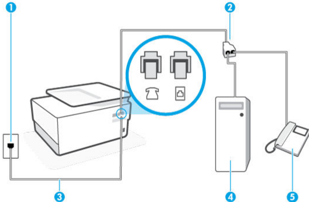
Kuva 8-9 Tulostin takaa
