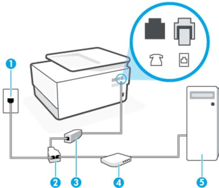
Kuva 8-7 Tulostin takaa
