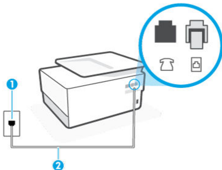
Kuva 10-2 Tulostin takaa
