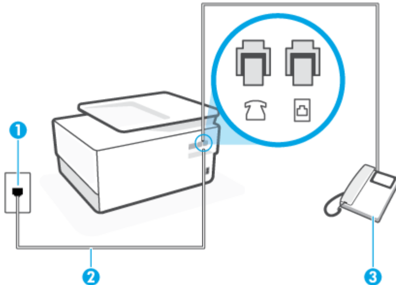
Kuva 8-4 Tulostin takaa
