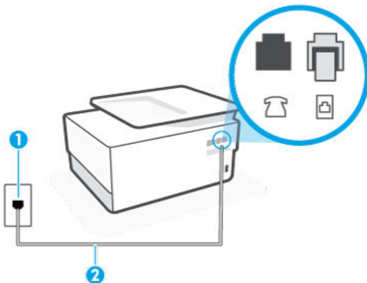
Rysunek 8-3 Widok drukarki z tyłu
