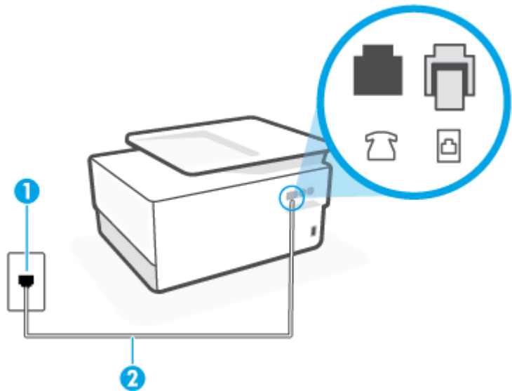
Figure 8-5 Vue arrière de l'imprimante
