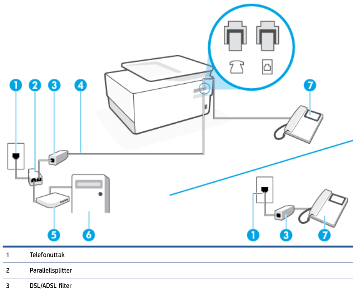
Figur 8-10 Skriveren sett bakfra
