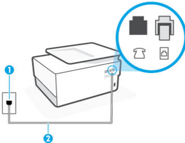
Figur 8-3 Skriveren sett bakfra
