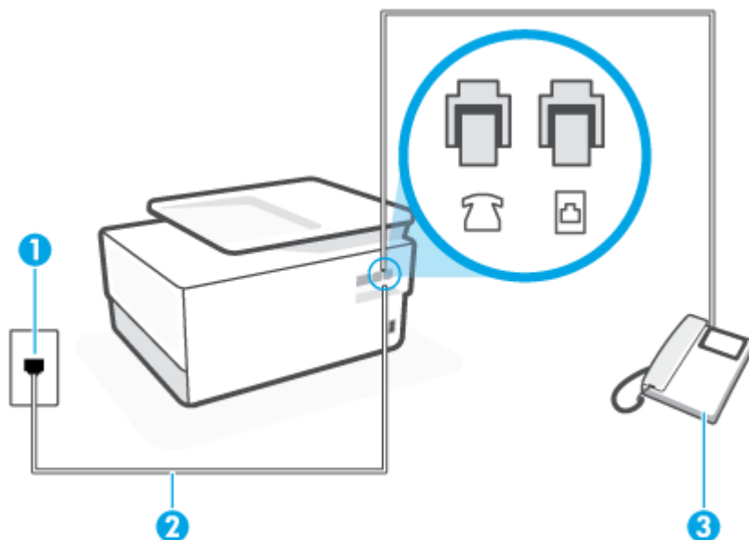
Фигура 8-4 Изглед на принтера отзад
