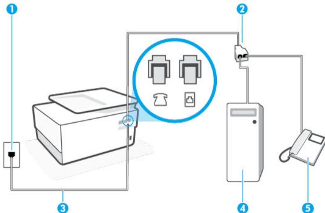
Фигура 8-9 Изглед на принтера отзад
