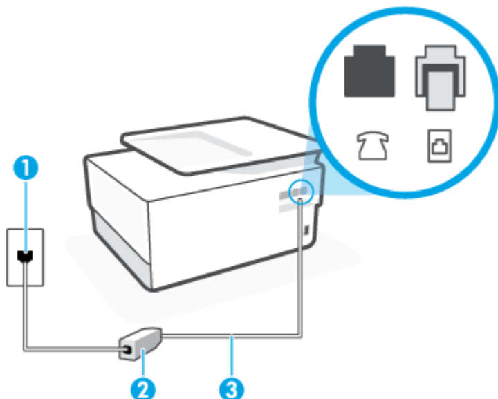
Фигура 8-2 Изглед на принтера отзад
