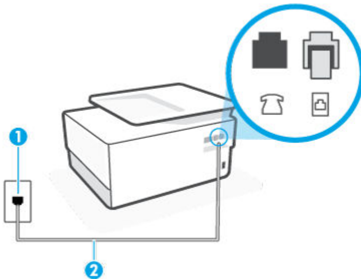
Фигура 8-5 Изглед на принтера отзад
