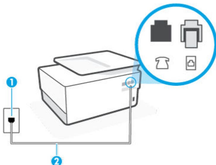
Figur 10-3 Skriveren sett bakfra
