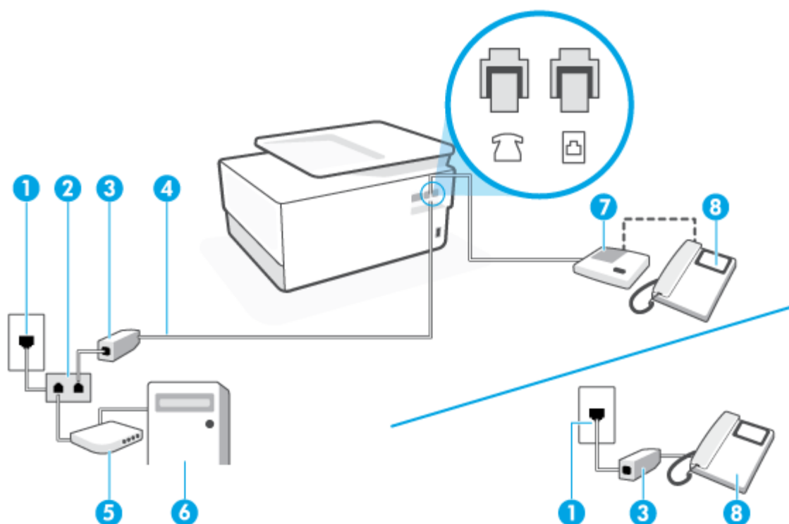
Figur 8-14 Skriveren sett bakfra
