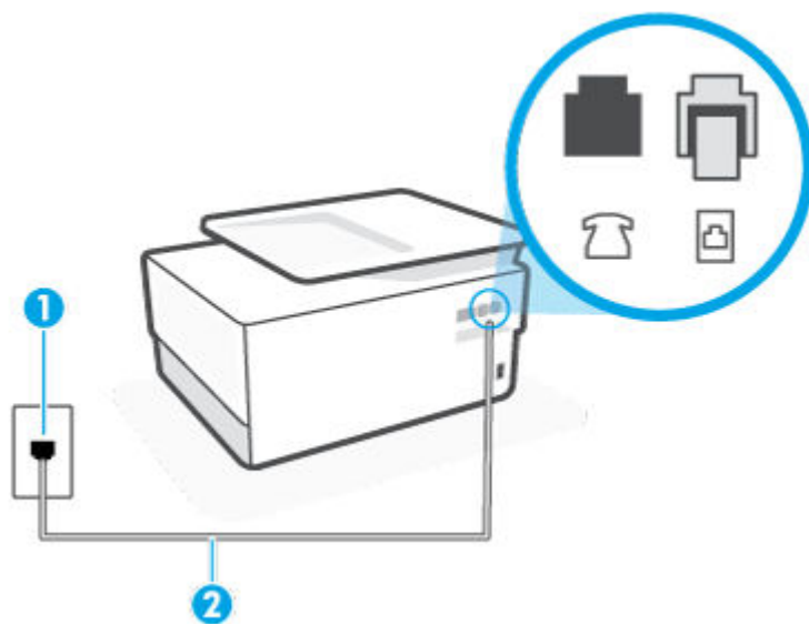
Figur 10-2 Skriveren sett bakfra
