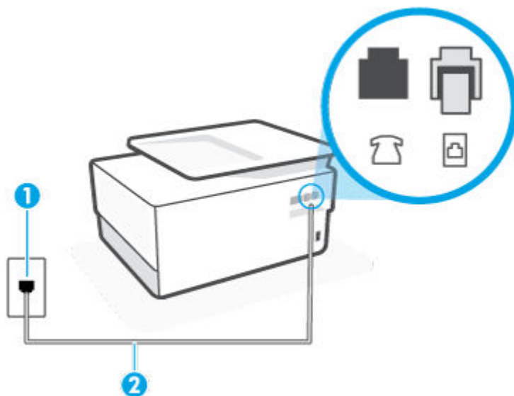
Bild 10-1 Skrivaren sedd bakifrån
