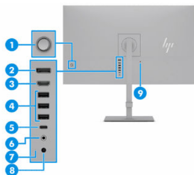
1-3. táblázat: A hátlap részegységei és azok leírása
