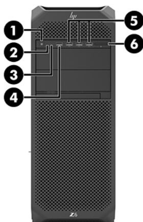
Tabuľka 2-4 Súčasti na prednej strane a ich opisy
