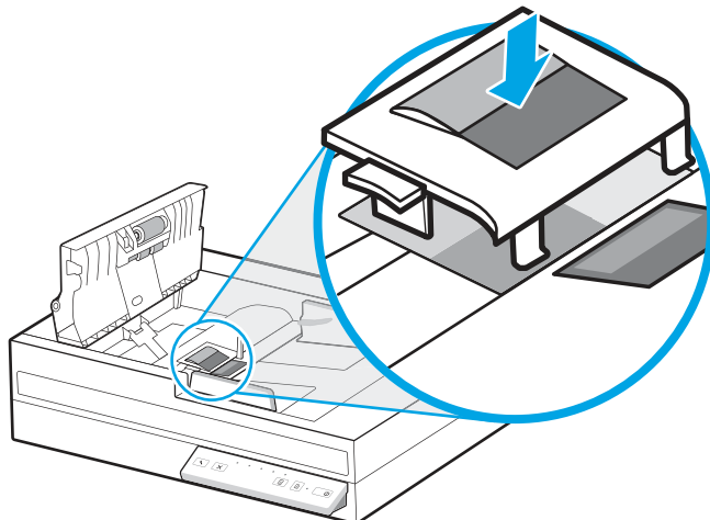
Εικόνα 3-4 Αντικατάσταση των κυλίνδρων διαχωρισμού (μοντέλα N4600 ffw1 και N6600 ffw1)
