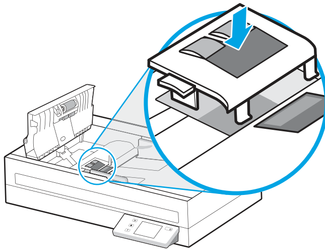
Εικόνα 3-4 Αντικατάσταση των κυλίνδρων διαχωρισμού (μοντέλα N4600 ffw1 και N6600 ffw1)
