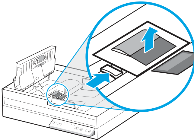
Εικόνα 3-1 Αφαίρεση του προστατευτικού διαχωρισμού (μοντέλα 2600 f1 και 3600 f1)
