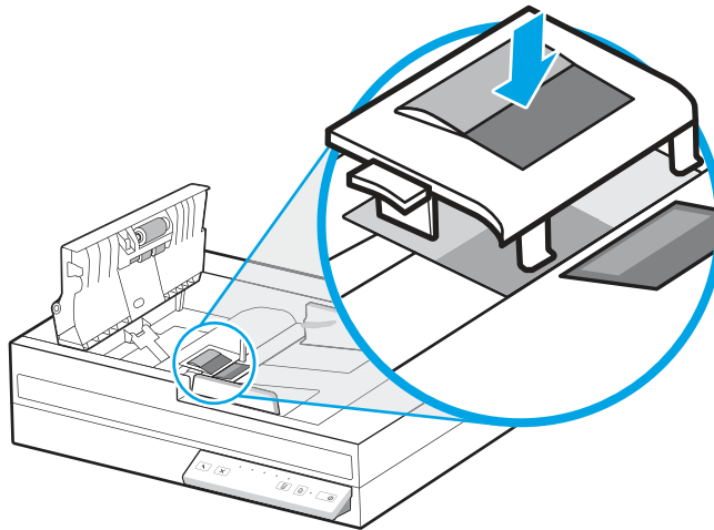
Gambar 3-4 Mengganti bantalan separasi (model N4600 fnw1 dan N6600 fnw1)
