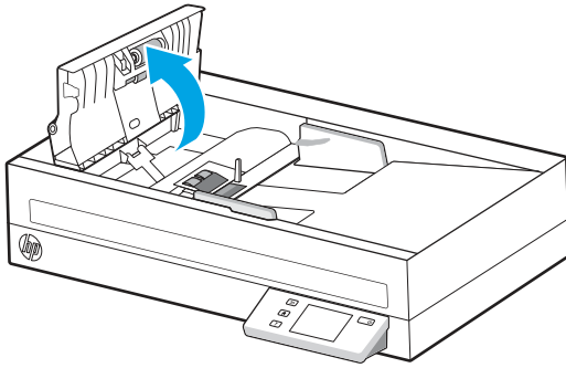
Gambar 3-1 Melepas bantalan separasi (model 2600 f1 dan 3600 f1)
