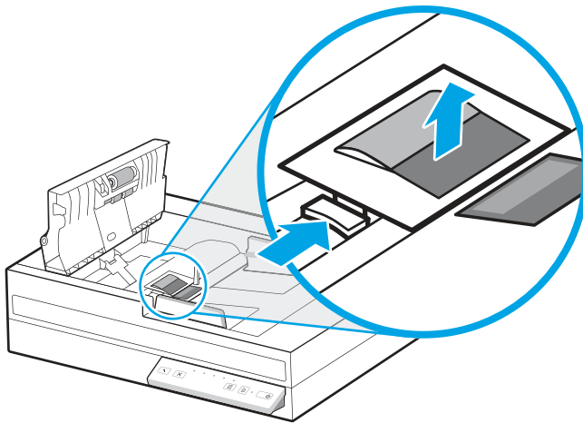
Gambar 3-2 Melepas rol separasi (model N4600 frw1 dan N6600 frw1)
