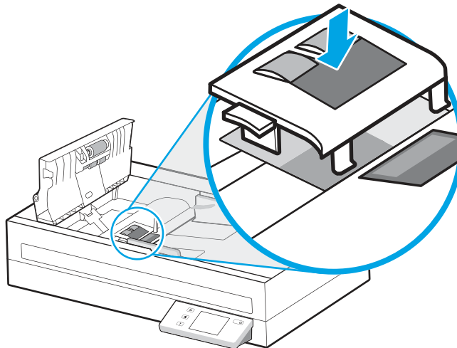
Gambar 3-4 Mengganti bantalan separasi (model N4600 fnw1 dan N6600 fnw1)
