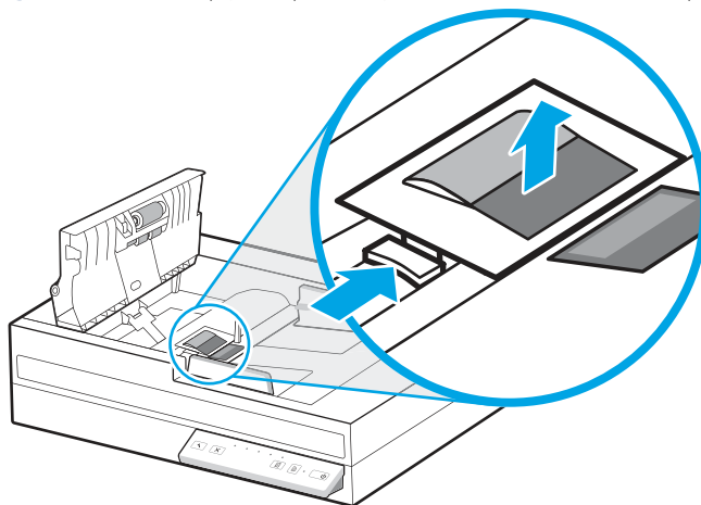
Figura 3-2 Scoateți rolele de separare (modelele N4600 fnw1 și N6600 fnw1)
