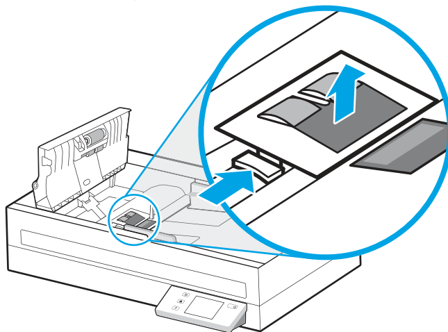
Figura 3-2 Scoateți rolele de separare (modelele N4600 fnw1 și N6600 fnw1)
