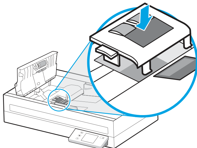
圖示 3-4 更換分紙滾筒 (N4600 fnw1 和 N6600 fnw1 機型)
