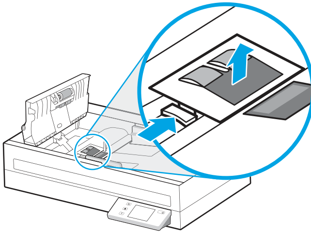
圖示 3-2 取出分紙滾筒 (N4600 fnw1 和 N6600 fnw1 機型)
