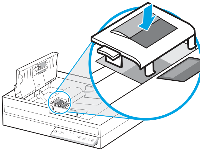
圖示 3-3 更換分隔墊 (2600 f1 和 3600 f1 機型)
