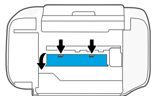
ด้านล่างของเครื่องพิมพ์
