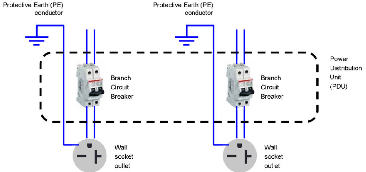
Abbildung 2-2 Elektrisches Konfigurationsdiagramm (nur zur Information)
