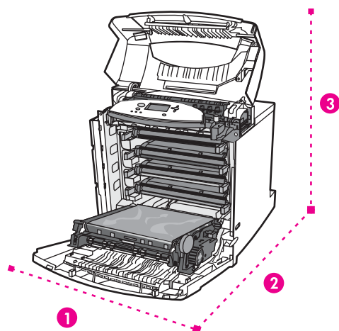
耗材更换空间示意图
