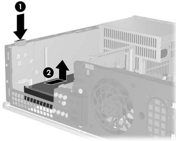
圖示 2-35 鬆開硬碟機
