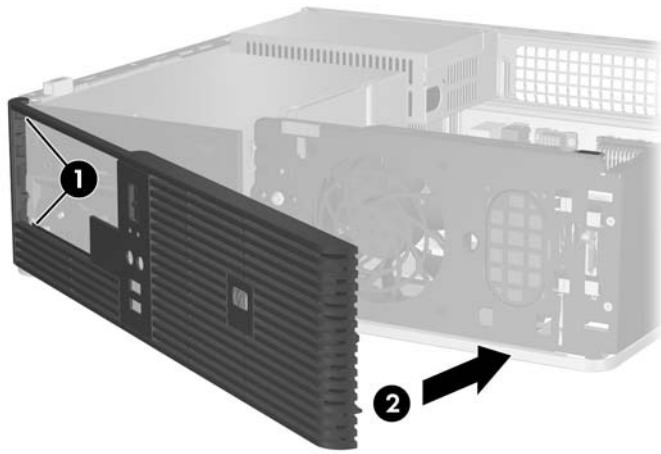
圖示 2-6 裝回正面機殼
