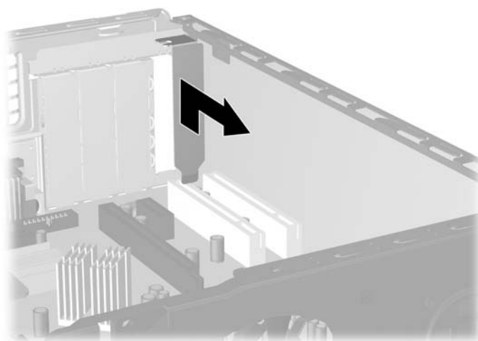
圖示 2-13 拆下擴充槽擋板
