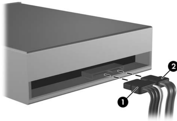
圖示 2-23 連接電源線和資料排線
