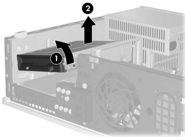
圖示 2-33 拆下軟碟機
