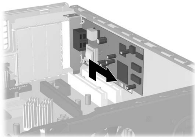
圖示 2-14 拆下標準 PCI 擴充卡
