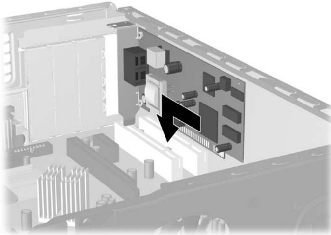
圖示 2-16 安裝擴充卡
