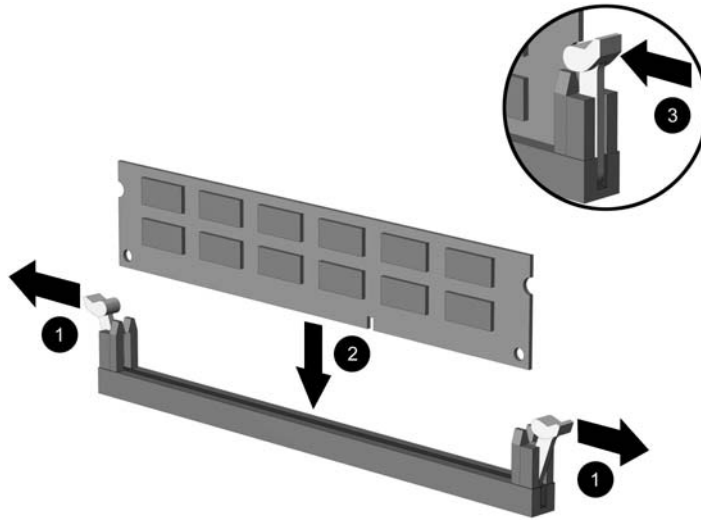
圖示 2-10 安裝 DIMM
