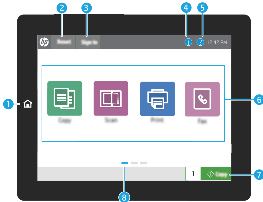
그림 1-4 제어판 보기
