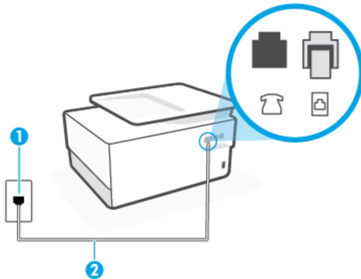
Abbildung 11-1 Rückansicht des Druckers
