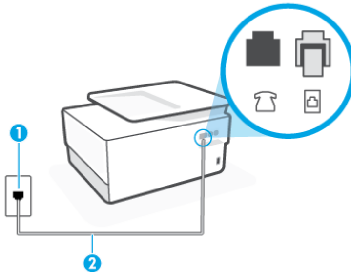
Abbildung 8-1 Rückansicht des Druckers
